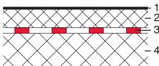
Schnitt Bodenaufbau 1 Bodenbelag 2 Unterlagsboden/Estrich 3 Elastische Bodenlagerung 4 Betondecke
